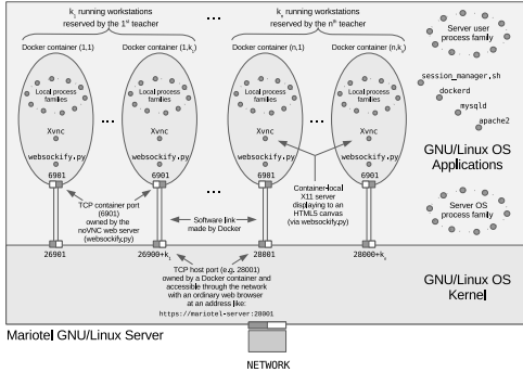
Fig. 3. Mariotel : Architecture logicielle
